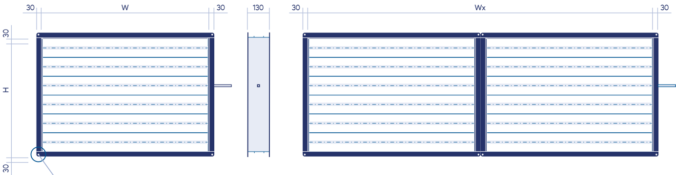
Stellachse mit Einkerbung zur Erkennung der Lamellenstellung
