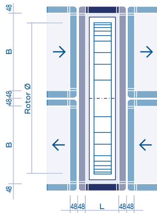
Draufsicht Luftströme nebeneinander
