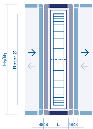
Draufsicht Luftströme übereinander mit Gehäuseverbreiterung / Seitenansicht Luftströme nebeneinander mit Gehäuseerhöhung
