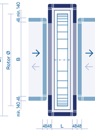
Draufsicht Luftströme übereinander Rotor zentriert
