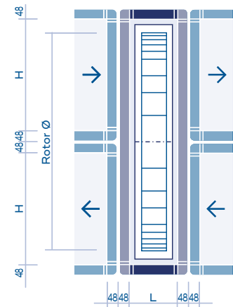
Seitenansicht Luftströme übereinander
